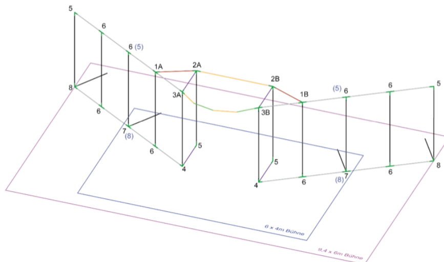
Gestänge, Aufbauplan M 1:50
